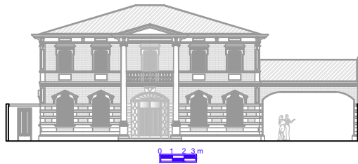
Elevation 01
