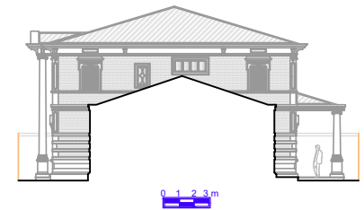
Elevation 04
